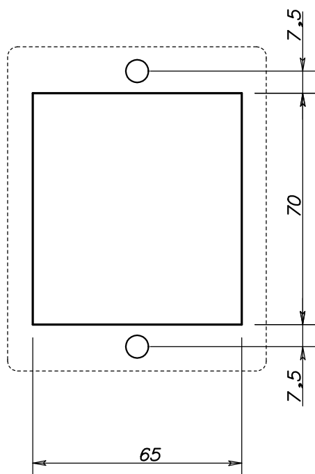
DIMENSIONI SCASSO
