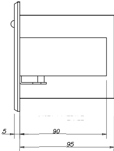
VUE DE COTE'
