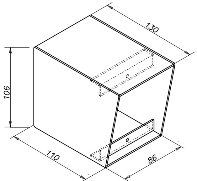
CARTER DE COUVERTURE REF 05651
