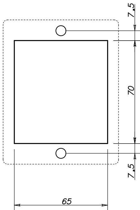
DIMENSIONI SCASSO
