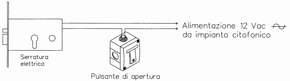
Collegamento serrature elettriche tradizionali
