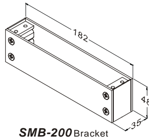
SMB-200 Bracket
